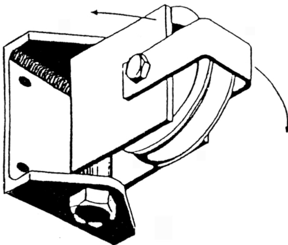
Umlenkrolle mit Konsole 520B-CO
