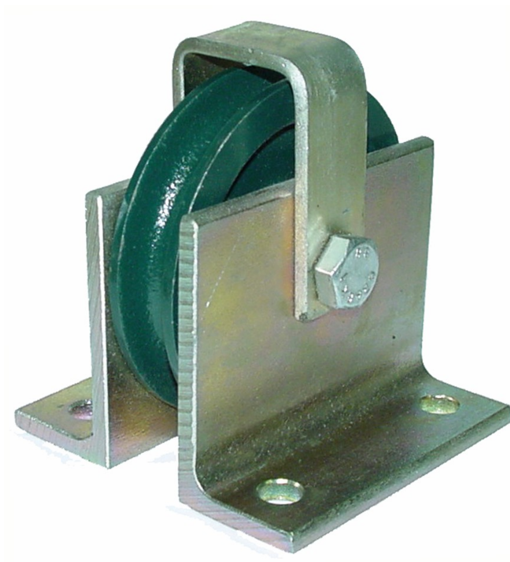
Seil-Umlenkrolle mit fester Konsole 837B-CO
