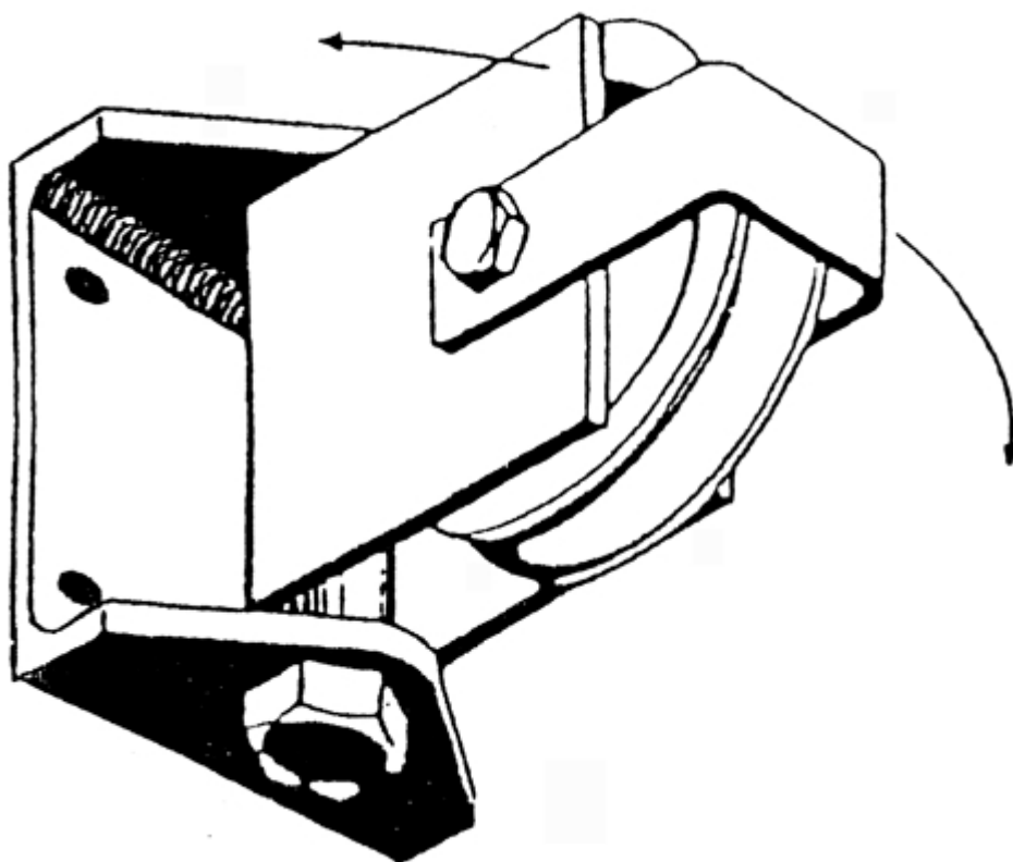
poulie de renvoi avec support 520B-CO
