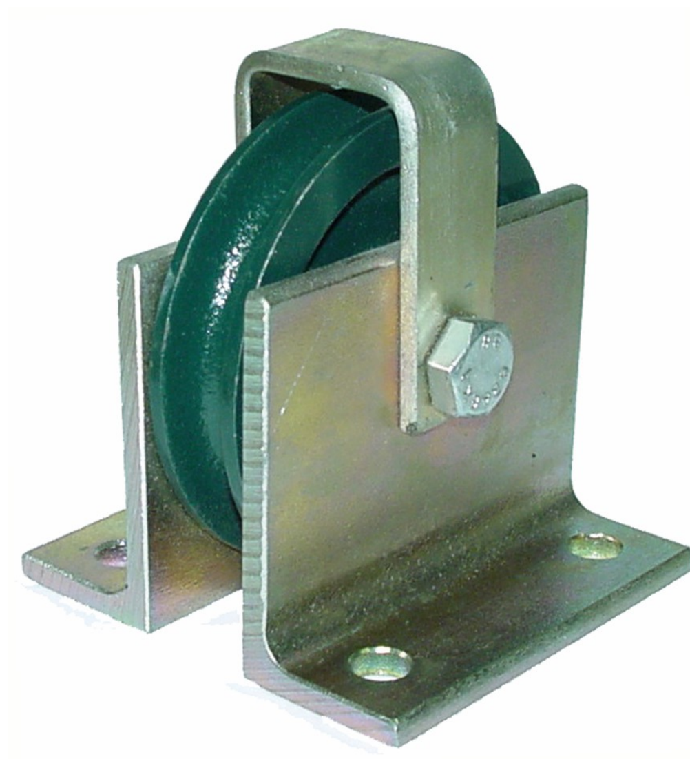
Poulie de renvoi pour câble en acier 837B-CO
